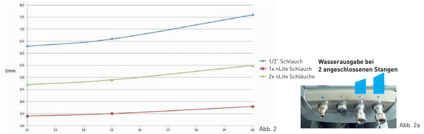
Abb. 2 Abhängigkeit der Leistung von Wassertemperatur und Schlauchdurchmesser bzw. Anzahl der Schläuche.
