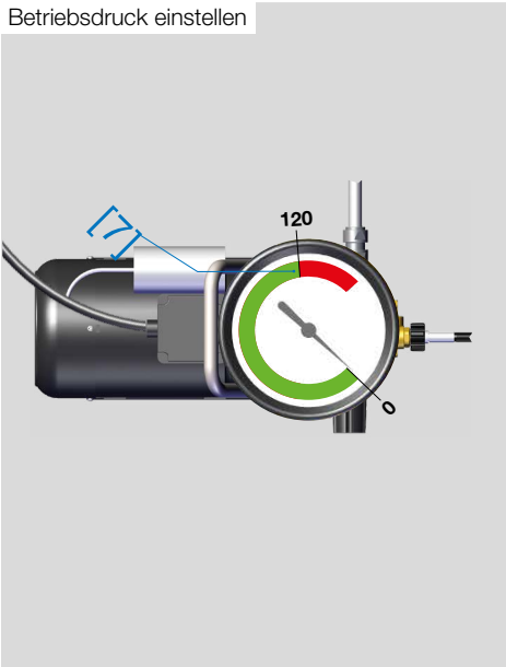
Betriebsdruck einstellen
