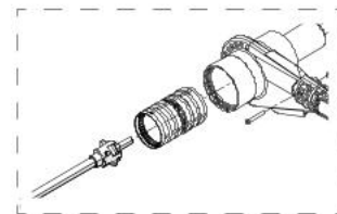
Montageposition der Scheiben. Assembly position of the washers
