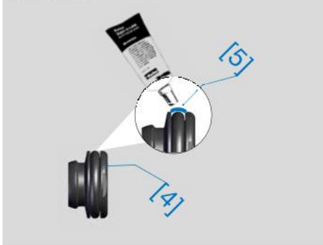
Lagereinheit auf Montagehilfe aufsetzen
